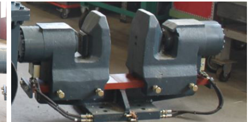
Klemmblock für Rohre Grand tube
